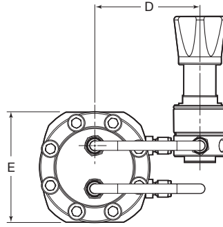
顶视图
