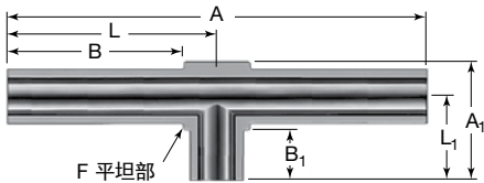
直通端加长三通接头
