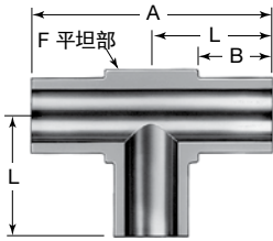
三通接头
