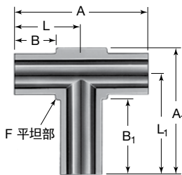
直通端加长三通接头
